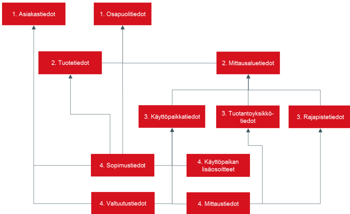
KUVA 4 SIIRTOTIEDOSTOJEN HIERARKIA.
